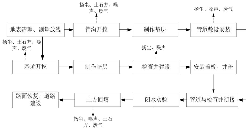
图 5-1 管网施工流程图示意图
