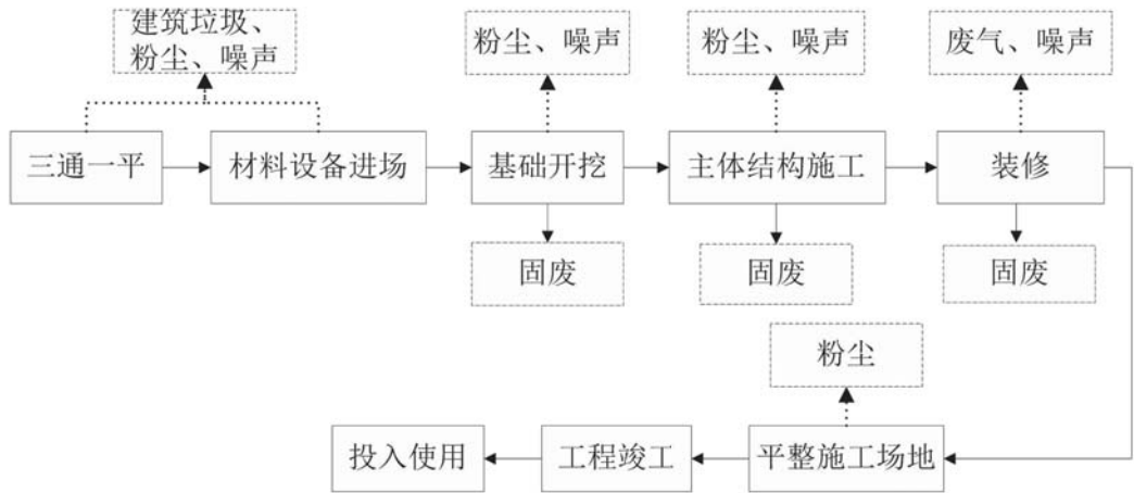
图 2 污水处理厂工程施工期工艺流程及产污环节图
