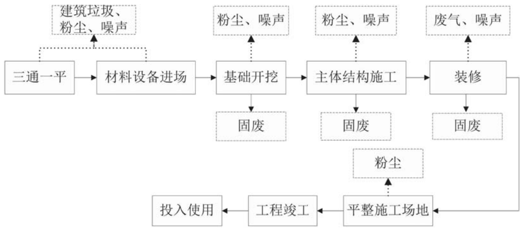
图 2 污水处理厂工程施工期工艺流程及产污环节图
