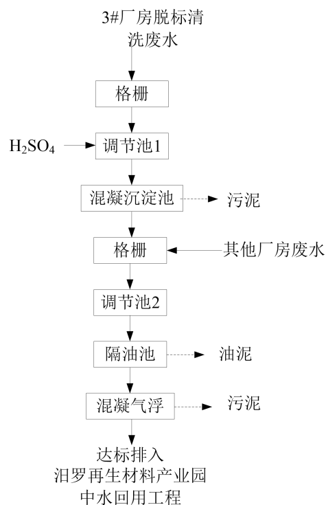
图 4-1 生产废水预处理流程图
