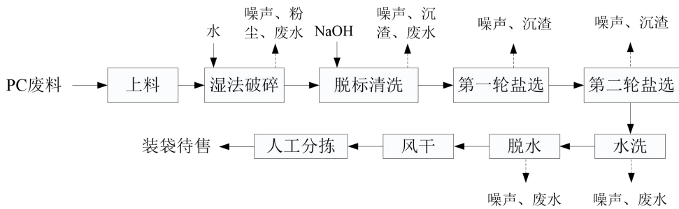
图 2-4 3#车间 PC 生产工艺流程图
