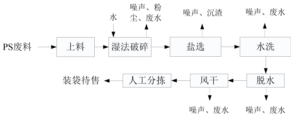
图 2-5 4#车间 PS 工艺流程图
