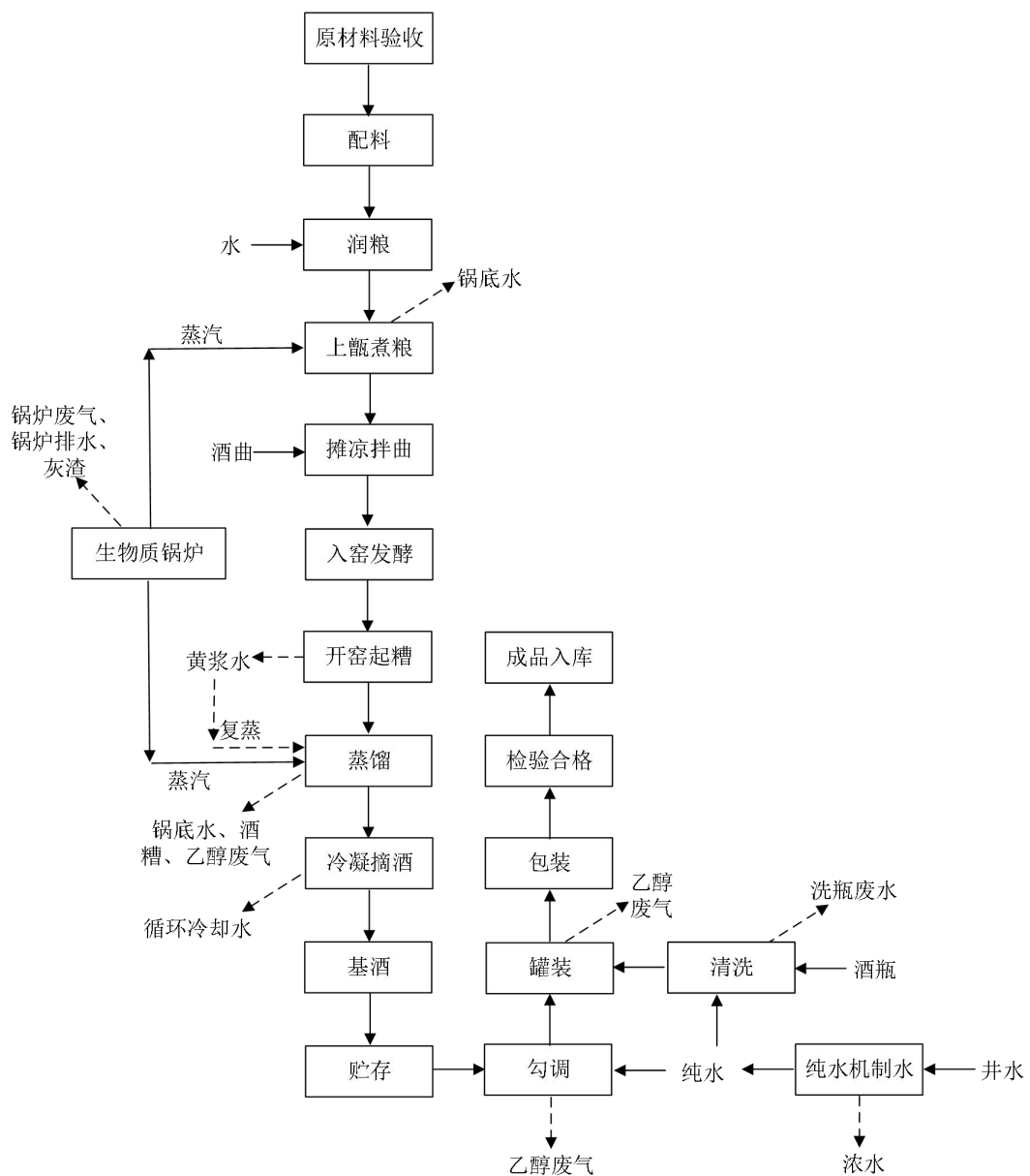
图 2-3 工艺流程和产污节点图
