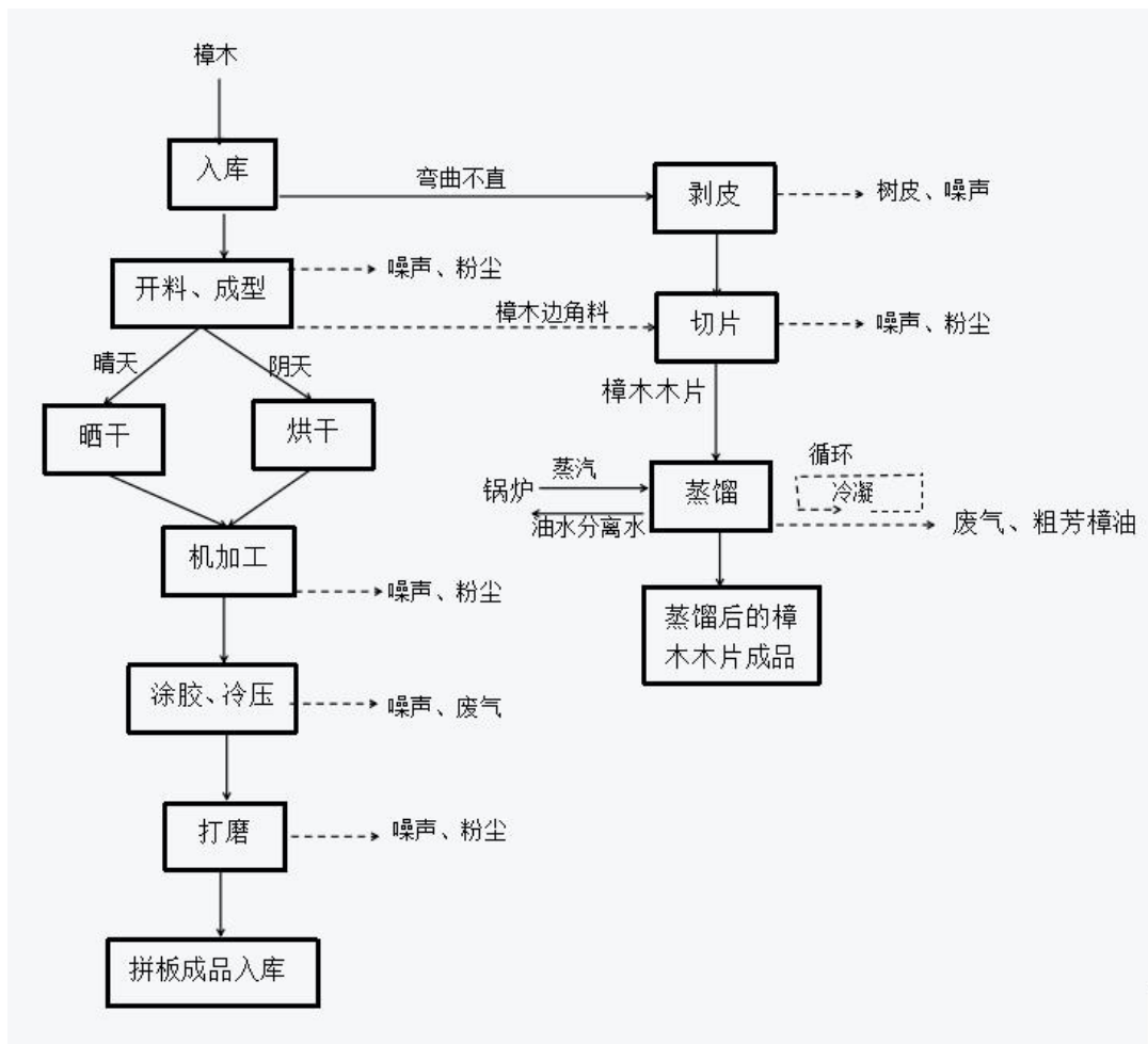
图 2-3 工艺流程图
